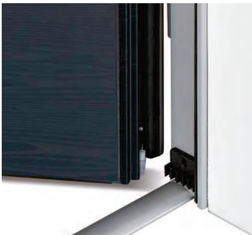
Particolare telaio a taglio termico con sistema a tripla guarnizione
