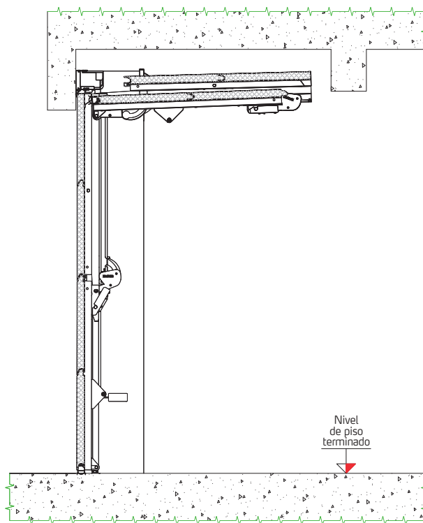
Garaje con obstáculos en el techo
