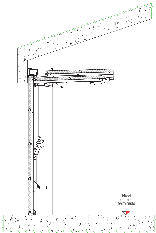
Garaje con techo inclinado
