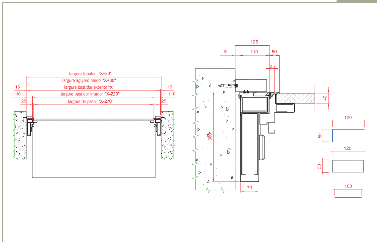
Sección horizontal - general
