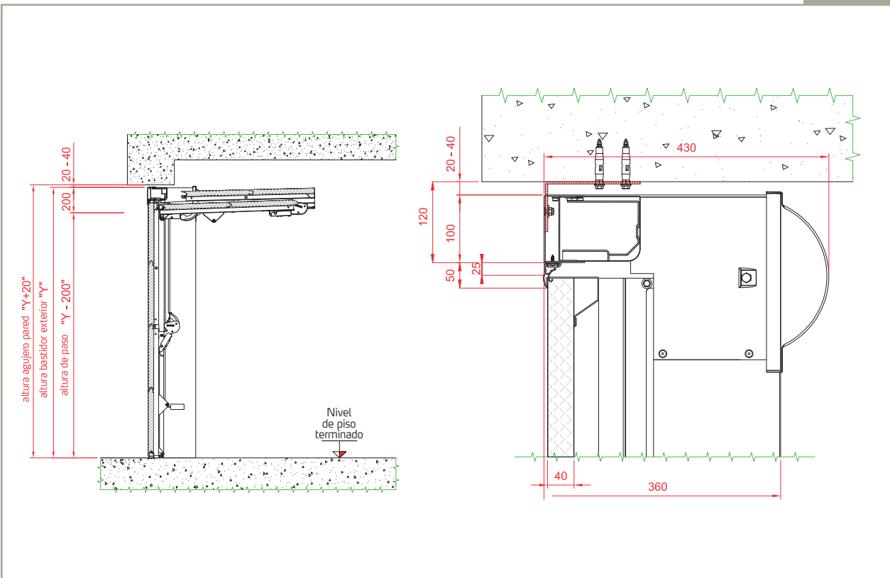
Sección vertical - general
