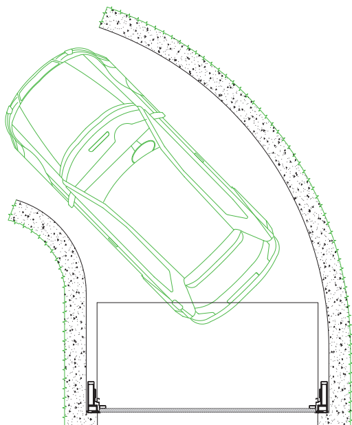
Garaje con paredes curvas
